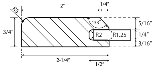
Shaker Door Profile
