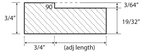
Slim Shaker Door Profile
